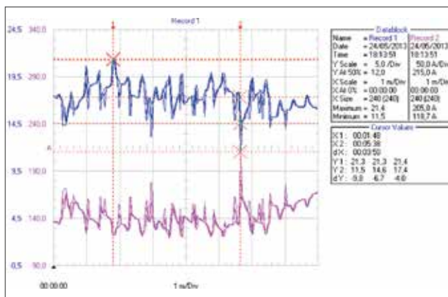
Figura 1. Forma de onda de corriente en CGBT típico.
