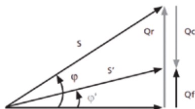
Figura 4. Ejemplo de compensación de factor de potencia. Representación vectorial.
