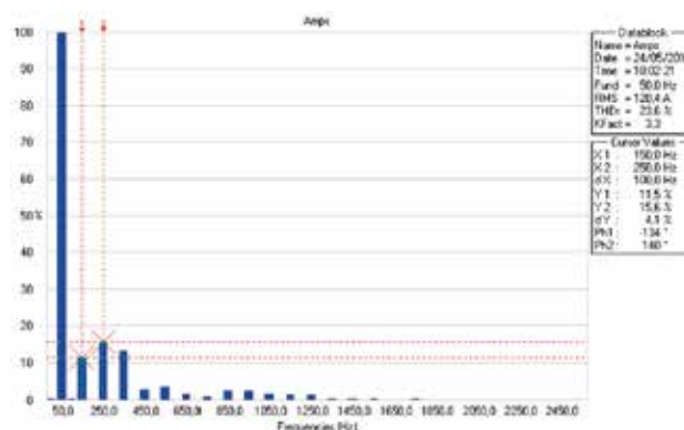
Figura 2. FFT de forma de onda de corriente en CGBT típico.
